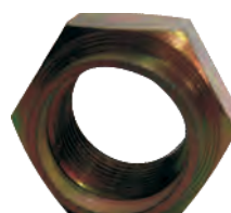
17195 CAJA MAZDA M24 X 1.5
